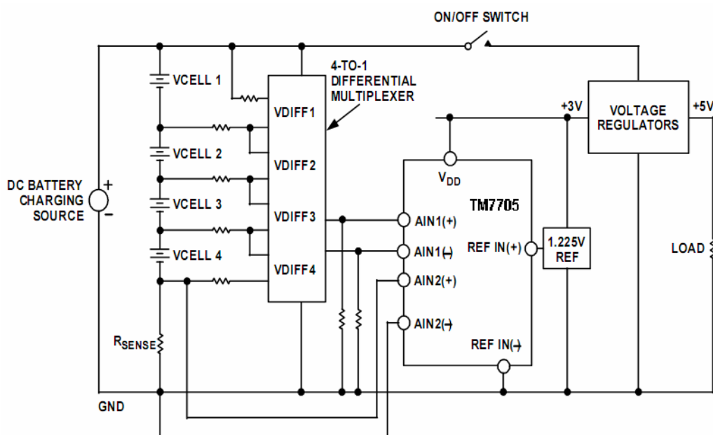
图 26 使用 TM7705 的电池监控电路
