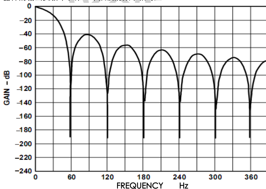
图 12 TM7705 滤波器的频率响应
