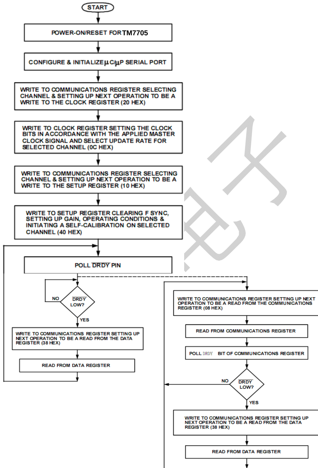
图 18 TM7705 的寄存器设置和读数流程图
