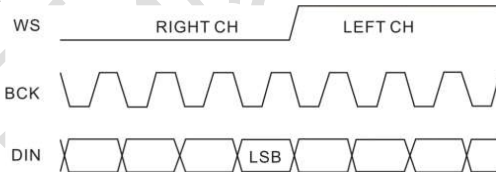
图1 信号输入格式
