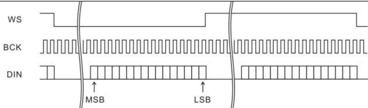
图2 信号输入时序
