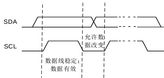
图 8.6 I 2 C 总线比特传输
