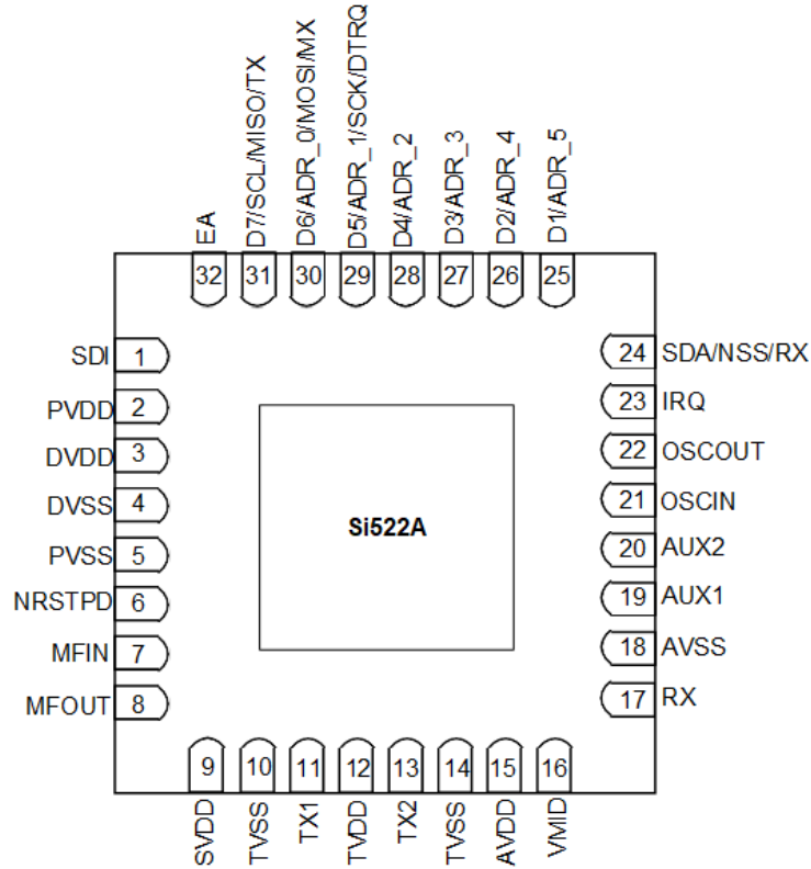
图 5.1 Si522A 管脚示意图
