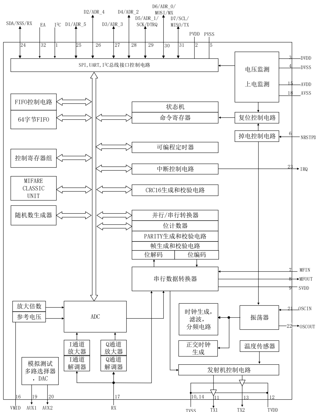
图 4.2 Si522A 功能框图
