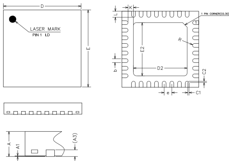
图 19.1 Si522A 封装示意图
