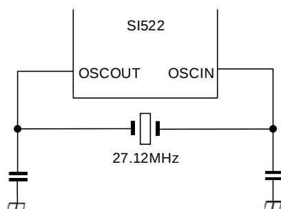
图 14.1 晶振连接
