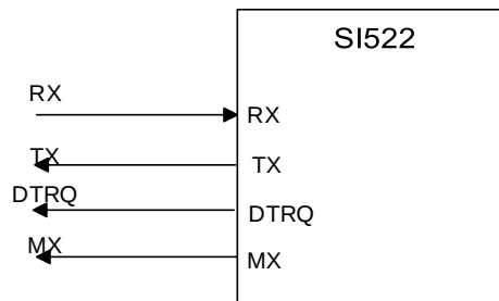
图 8.2 UART 接口
