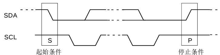
图 8.7 起始和停止条件
