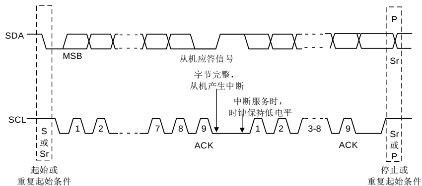
图 8.9 I²C 总线数据传输示意图
