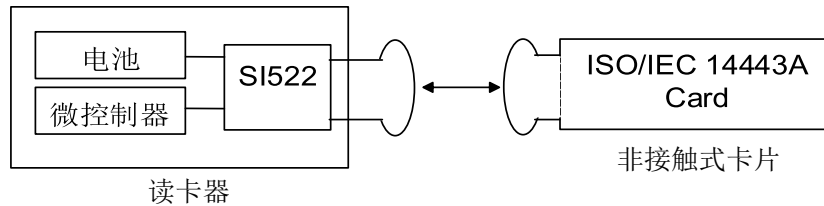
图 6.1 Si522A 读卡模式
