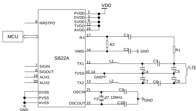
图 17.1 Si522A 典型应用电路图
