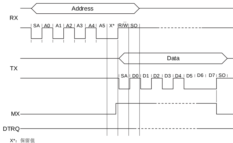
图 8.3 UART 读数据时序图
