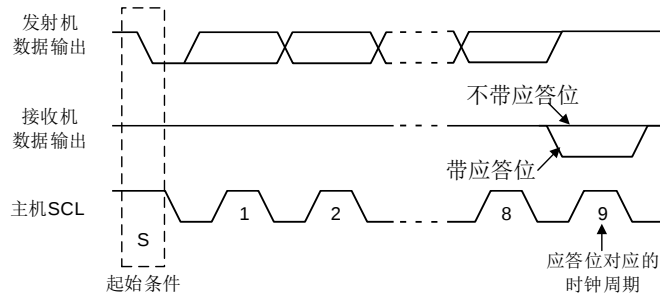
图 8.8 I²C 总线应答位
